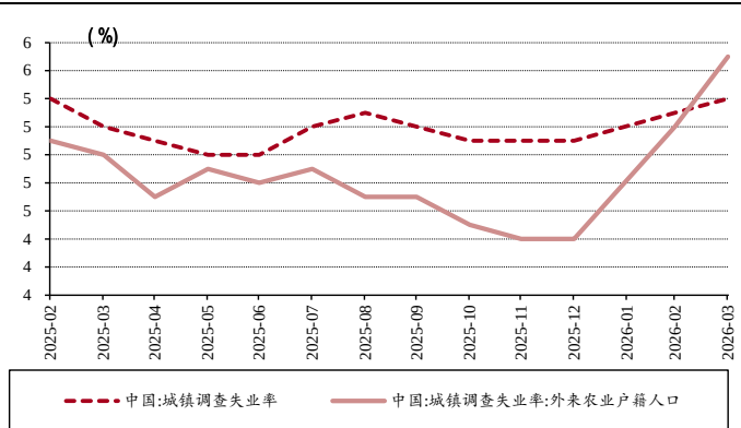
图表 3. 失业率数据表现
